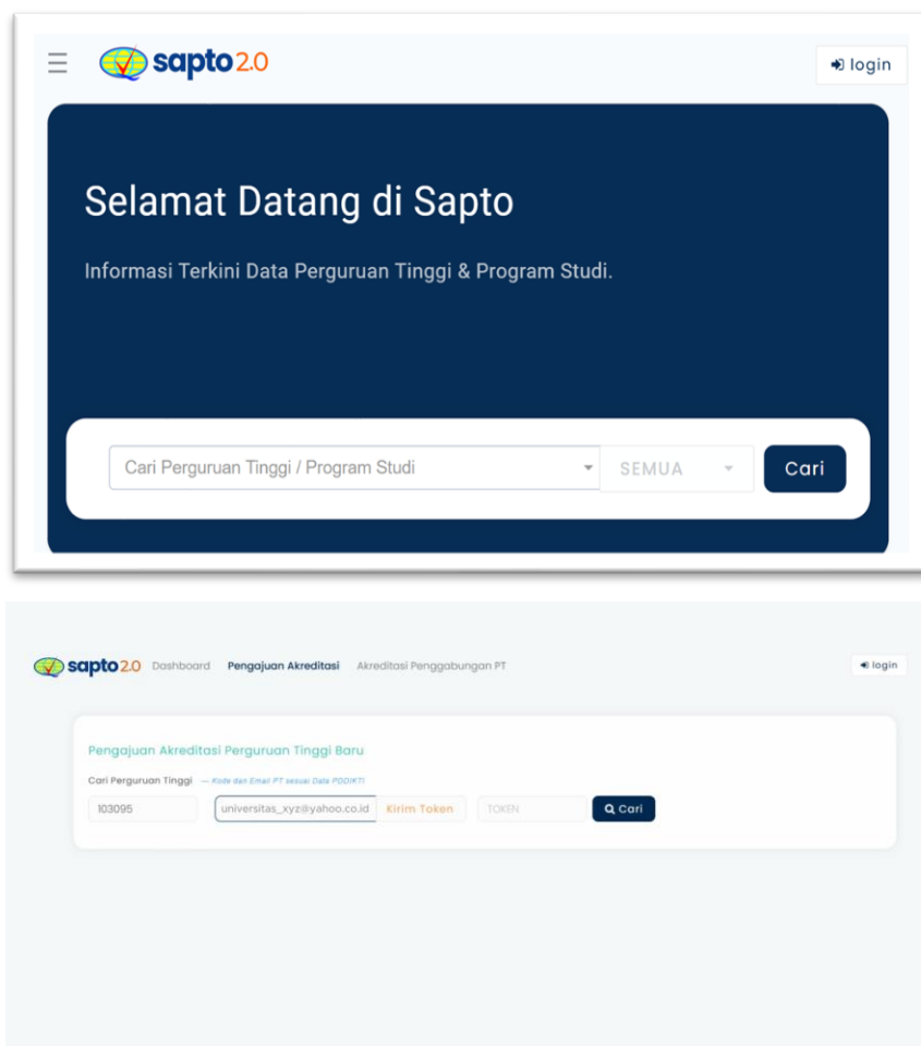
Gambar 8. Tampilan SAPTO 2.0
